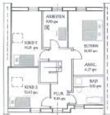
Grundriss Obergeschoss
