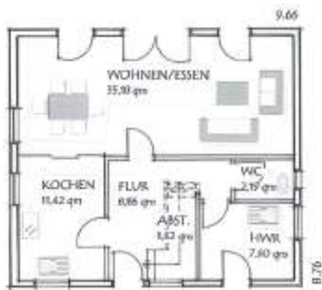
Grundriss Erdgeschoss
